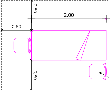
SCHEMA TIPO POSTO LETTO Sedia/sgabello
